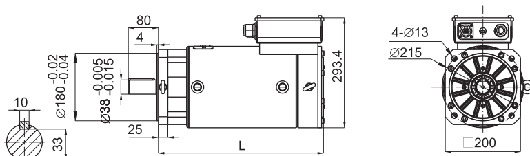
200机座安装尺寸示意图
