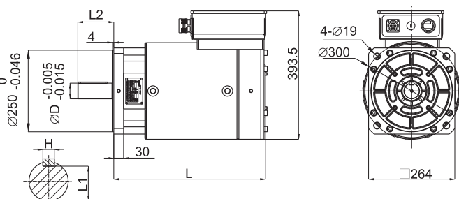
260机座安装尺寸示意图
