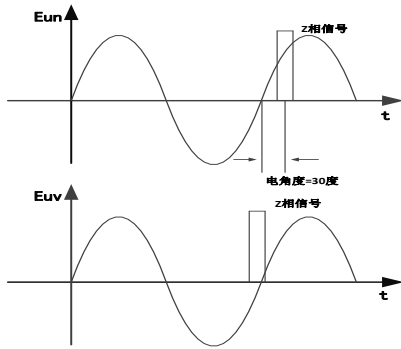
图 4-14a Z 相信号位置定义
