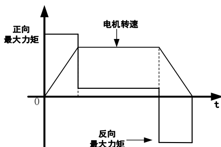
图 6-8c 无力矩限制图
