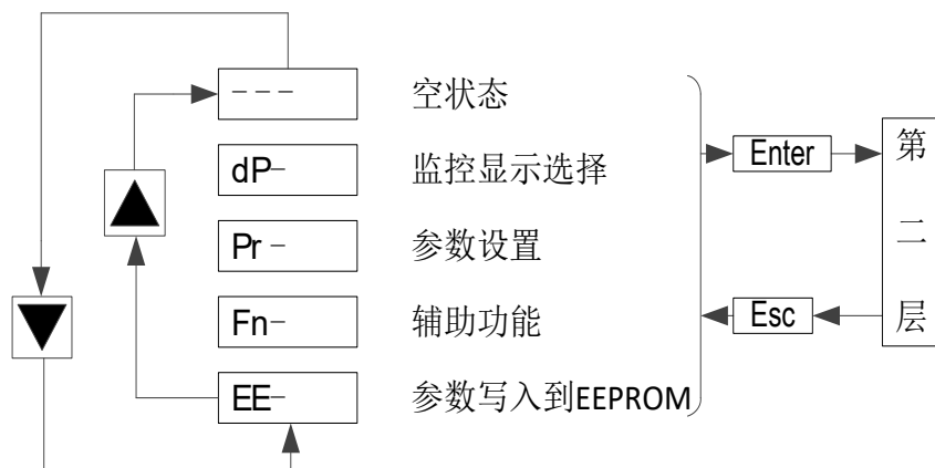
图 5-2 第一层主菜单框图
