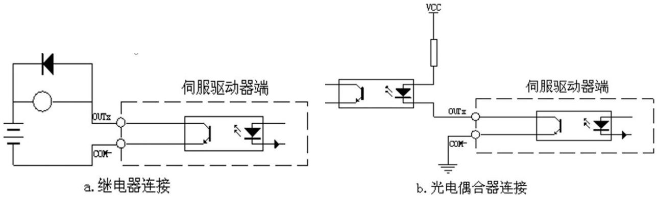
图 4-10 典型数字输出端口应用
