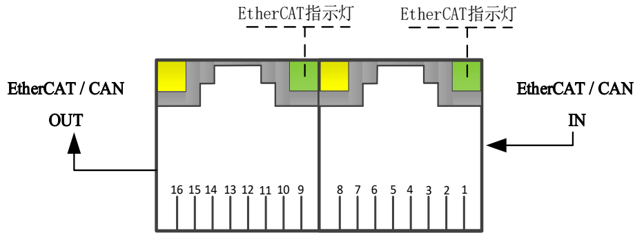
图 4-8 以太网或者 CAN 接口（面对插口看）
