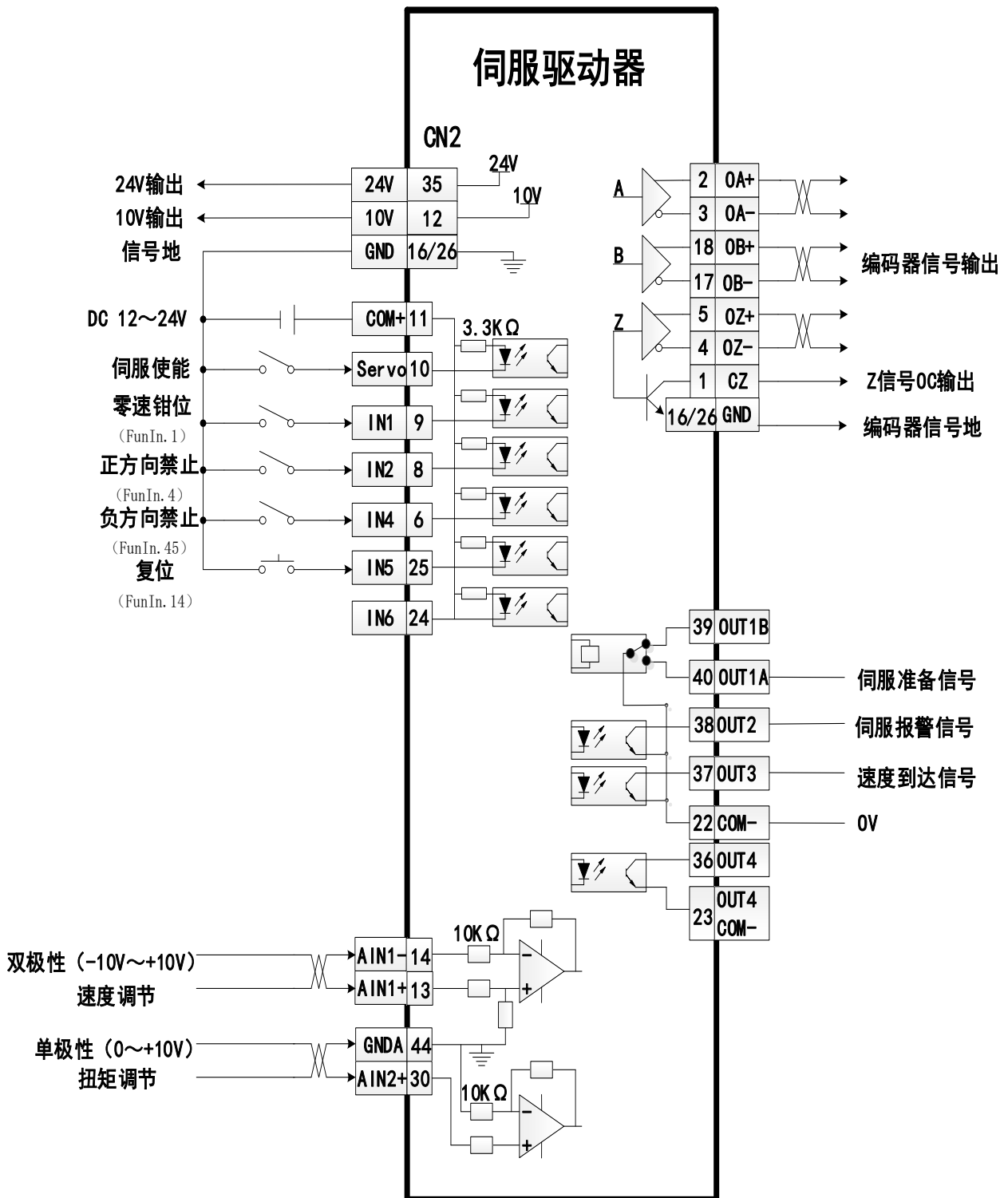
图 6.9 力矩限制（单极性）模式下 CN2 的简易接线图
