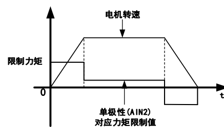
图 6-8d 内部力矩限制图
