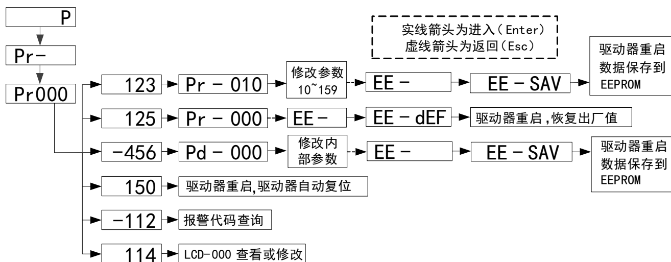
图 5-11 密码操作示意图
