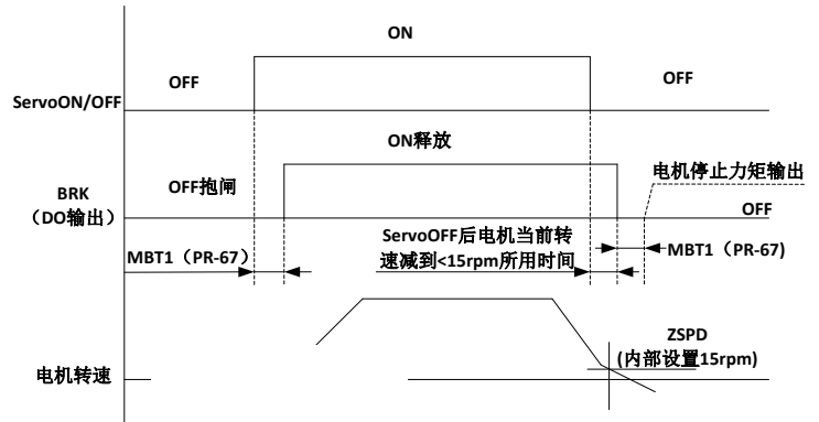
图6-2 制动器的控制时序
