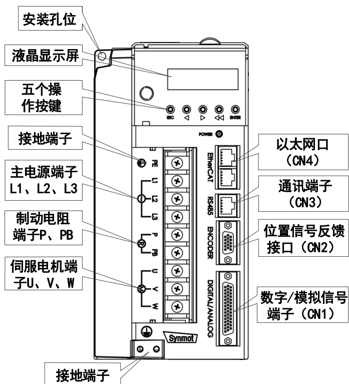
图2.1 SM30 系列 11kW以下（书本式）
