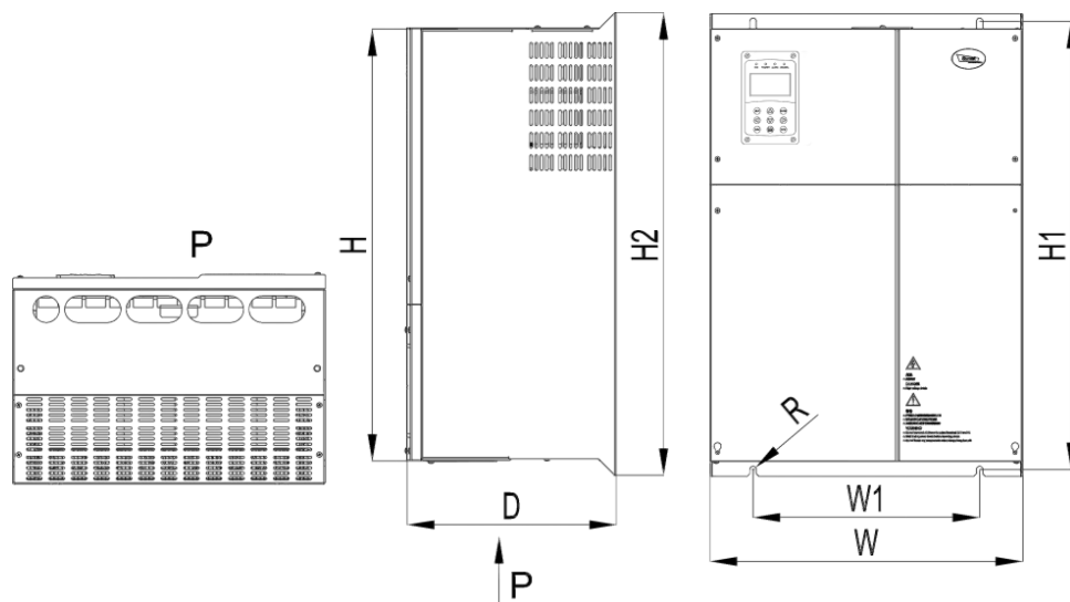
图 3-3 SM30 系列 11kW~160kW 安装及外形尺寸示意图
