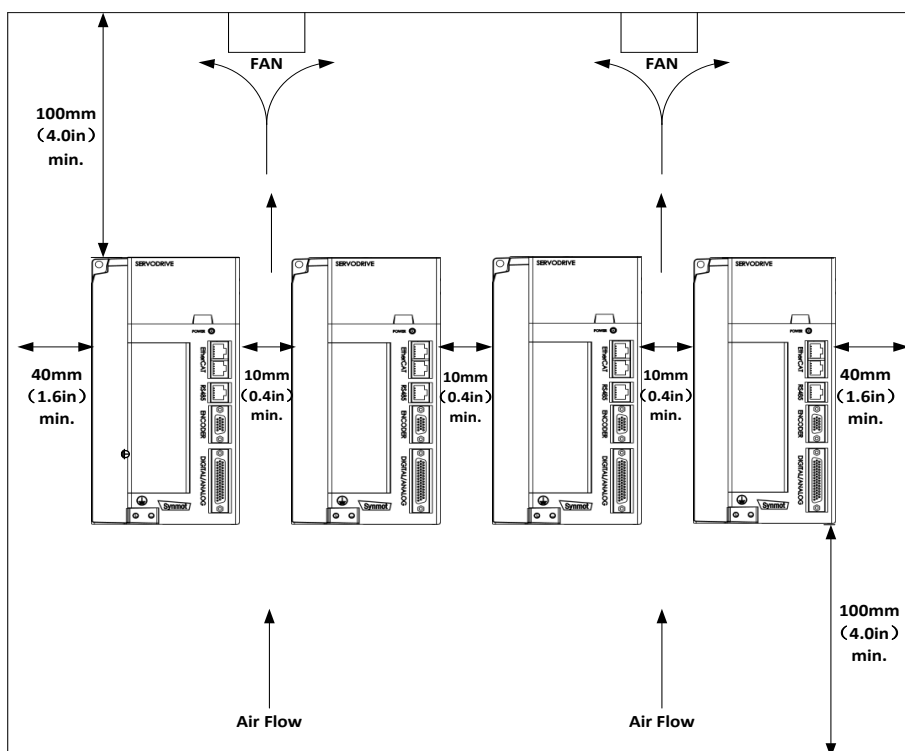
图 3-5 多台驱动器的安装间隔
