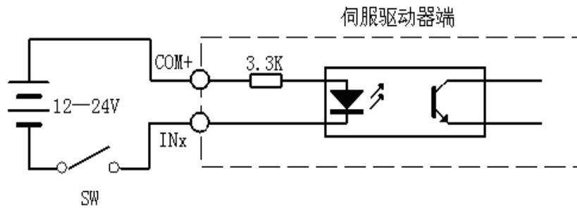
图 4-9 数字输入接口
