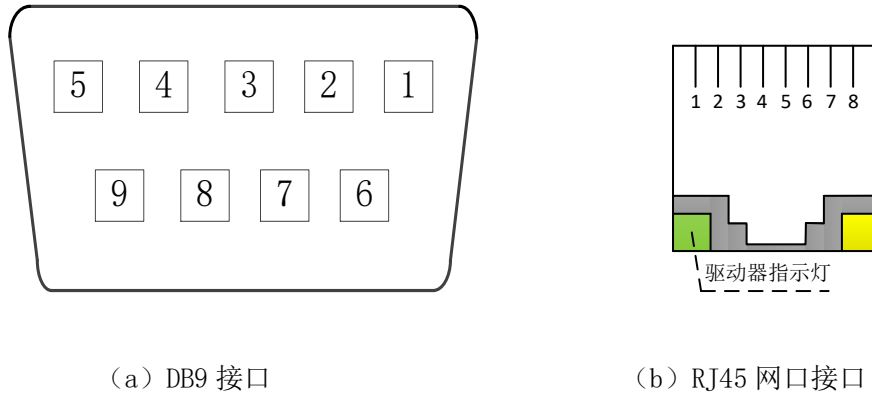
图 4-7 RS485/CAN 通讯插头
