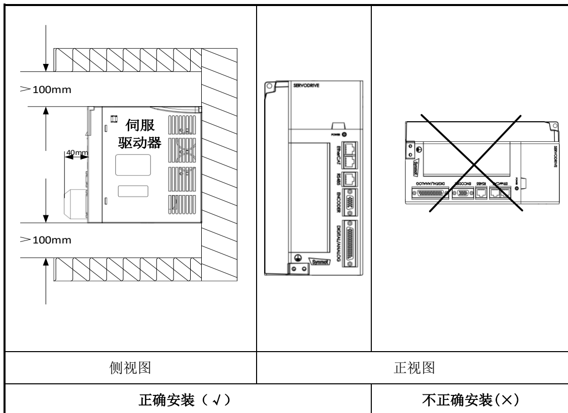
图 3-3 驱动器基座安装方式图
