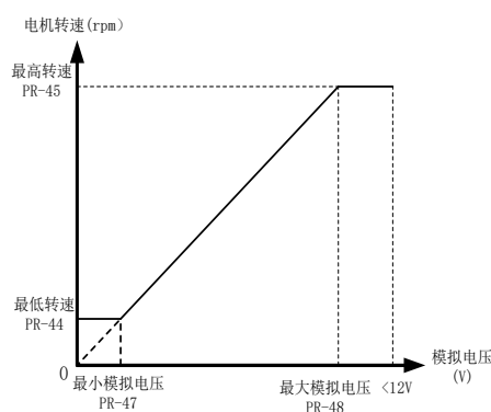
图6-5b 单极性信号输入与电机转速比例图
