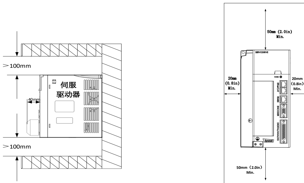
图 3-4 单台驱动器的安装间隔
