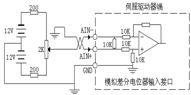
图 4-11d 模拟双极性单端输入接口 电压范围 -10V~+10V
