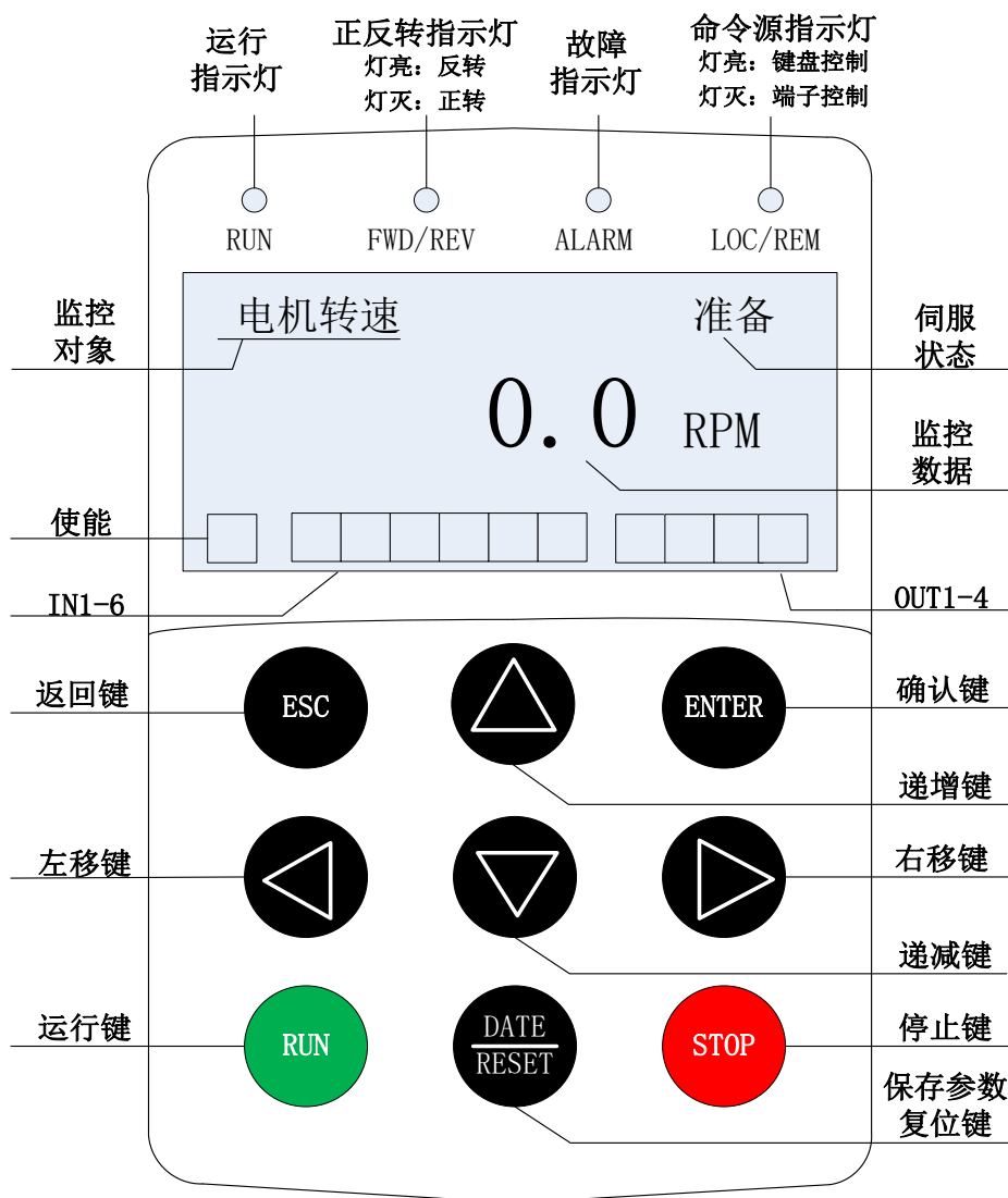
图 5-10 LCD 操作面板外观图
