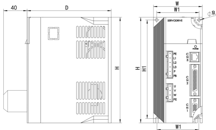
图 3-1 SM30 系列款式 A 尺寸示意图
