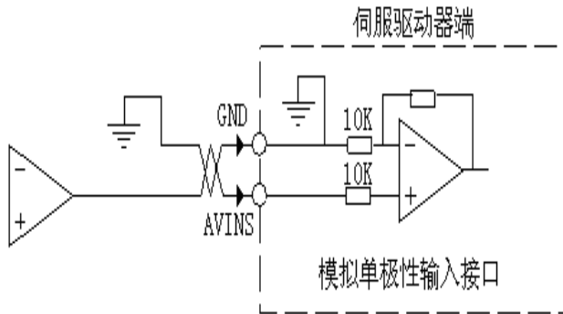
图 4-11a 模拟单极性输入接口 电压范围 0~+10V
