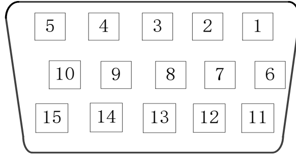
图 4-5 位置反馈插头 DB15
