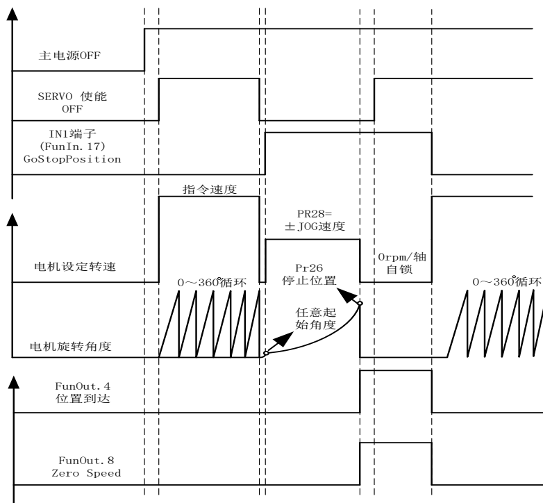
图 6-7 定向控制时序图
