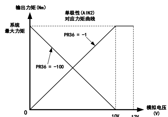
图 6-8b AIN2 外部指令与力矩限制关系图
