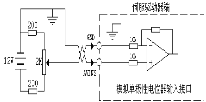
图 4-11b 模拟单极性电位器输入接口 电压范围 0~+10V
