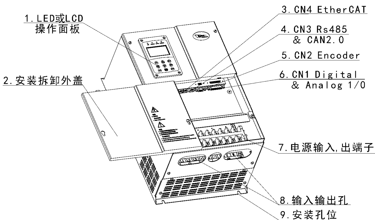
图2.2 SM30 系列 11kW以上（箱体式）
