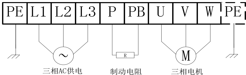
图 4-4A 11kW（含）以下驱动器主回路端子示意图（书本式）
