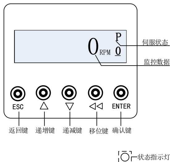
图 5-10 LCD 操作面板外观图
