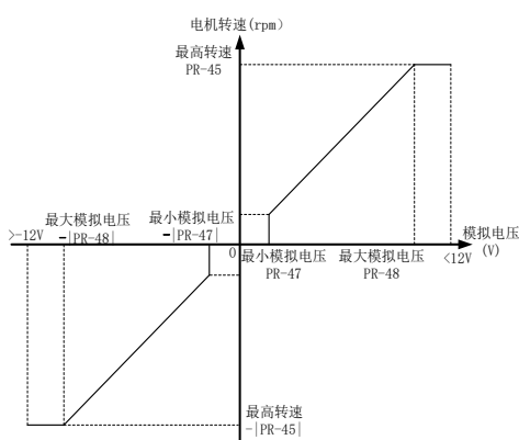
图6-5a 双极性信号输入与电机转速比例图
