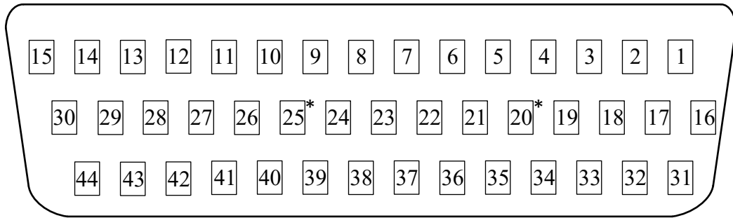
图 4-6 数字/模拟信号端子插头 DB44
