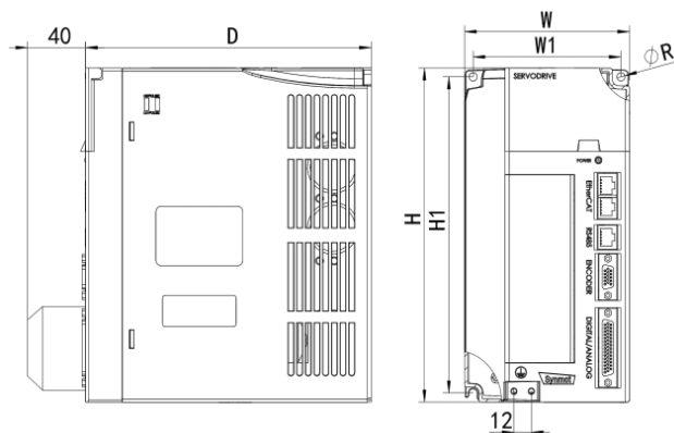
图 3-2 SM30 系列款式 B 尺寸示意图
