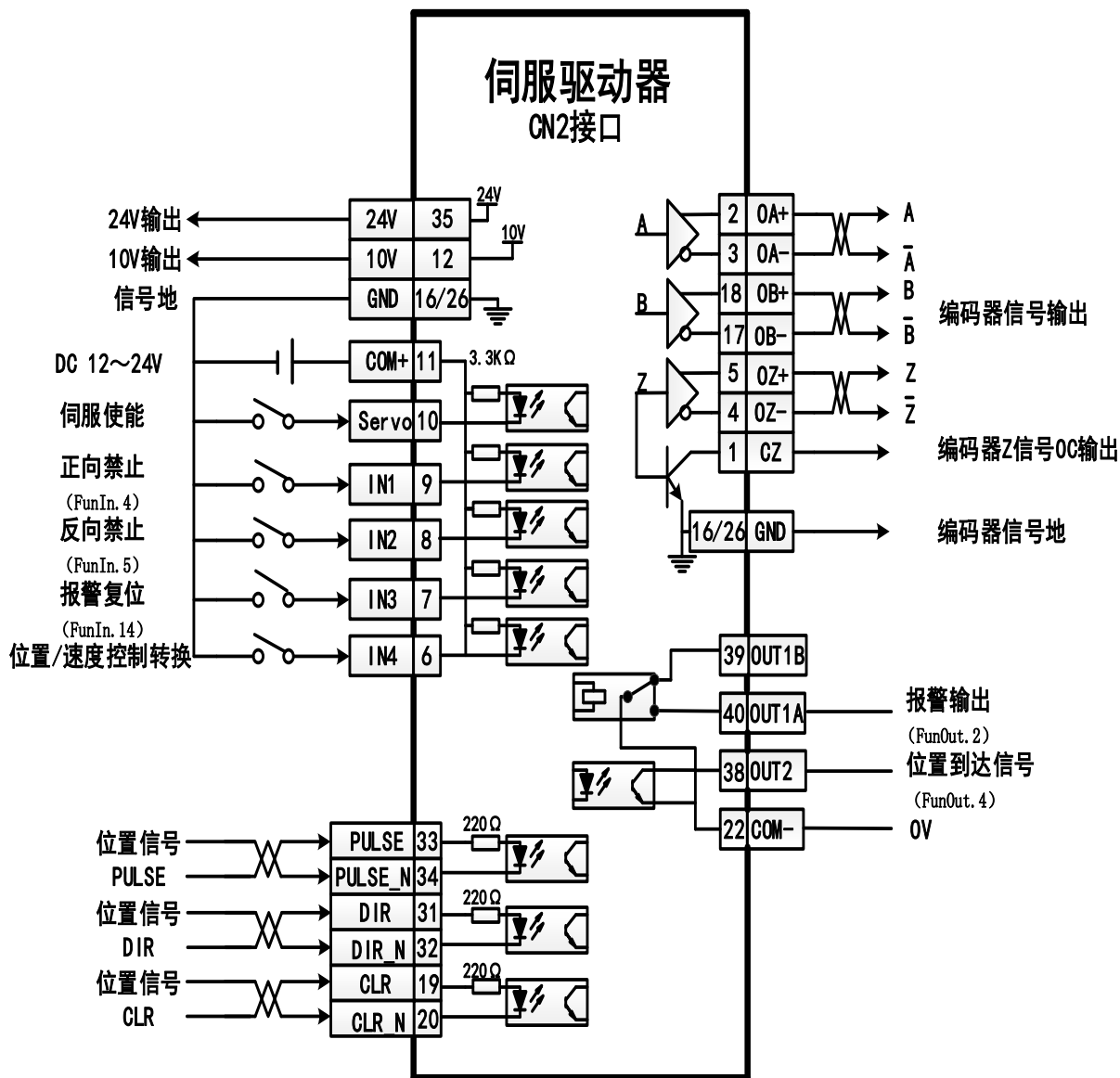
图6-4 位置控制方式下CN2的简易接线图
