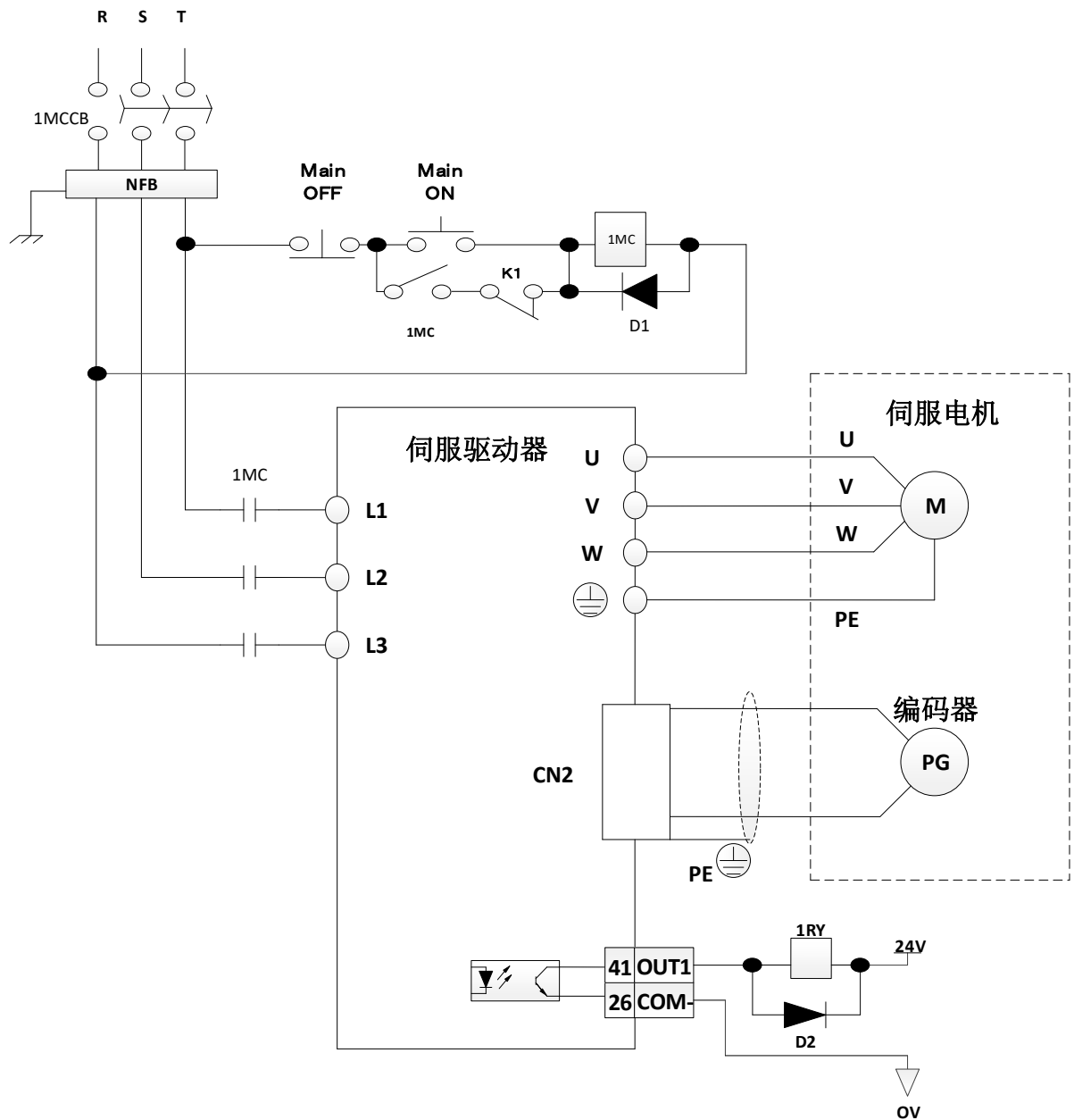
图 4-2 主电源接线图
