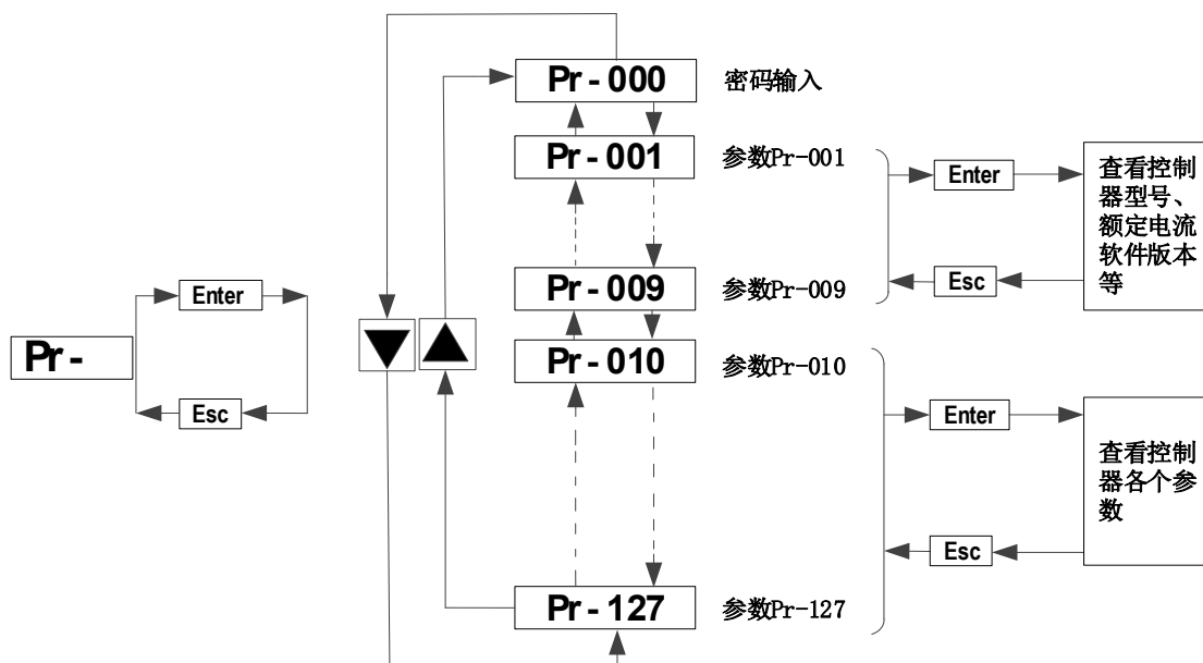
图 5-4 参数设置
