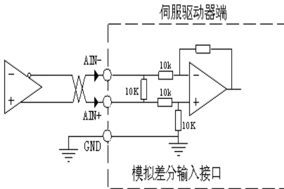
图 4-11c 模拟双极性差分输入接口 电压范围差分 -5V~+5V
